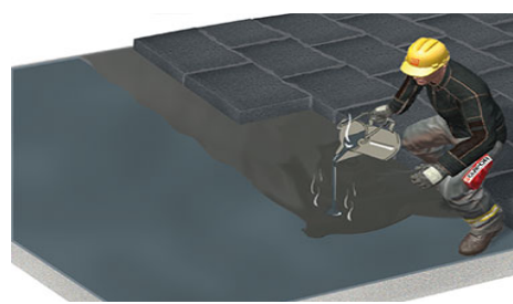
Heißbitumen verteilen
