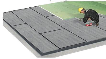
XPS-Zusatzdämmung verlegen
