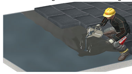
Platten vollflächig in Heißbitumen verlegen
