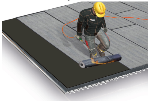
bituminöse Abdichtung herstellen
