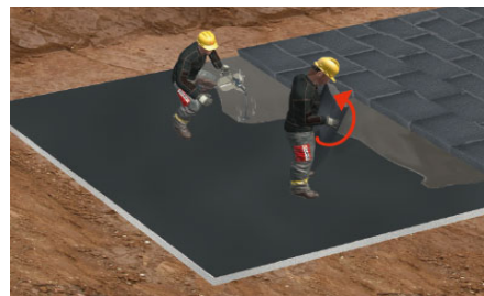
GLAPOR Schaumglasplatten in Heißbitumen
